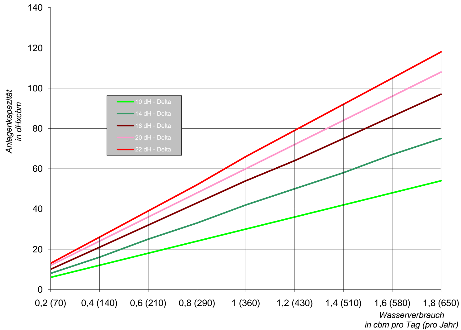
Notwendige Anlagenkapazität in Abhängigkeit zum Wasserverbrauch und gewünschter Enthärtung Delta (Rohwasserhärte - Zielhärte) des Wassers
